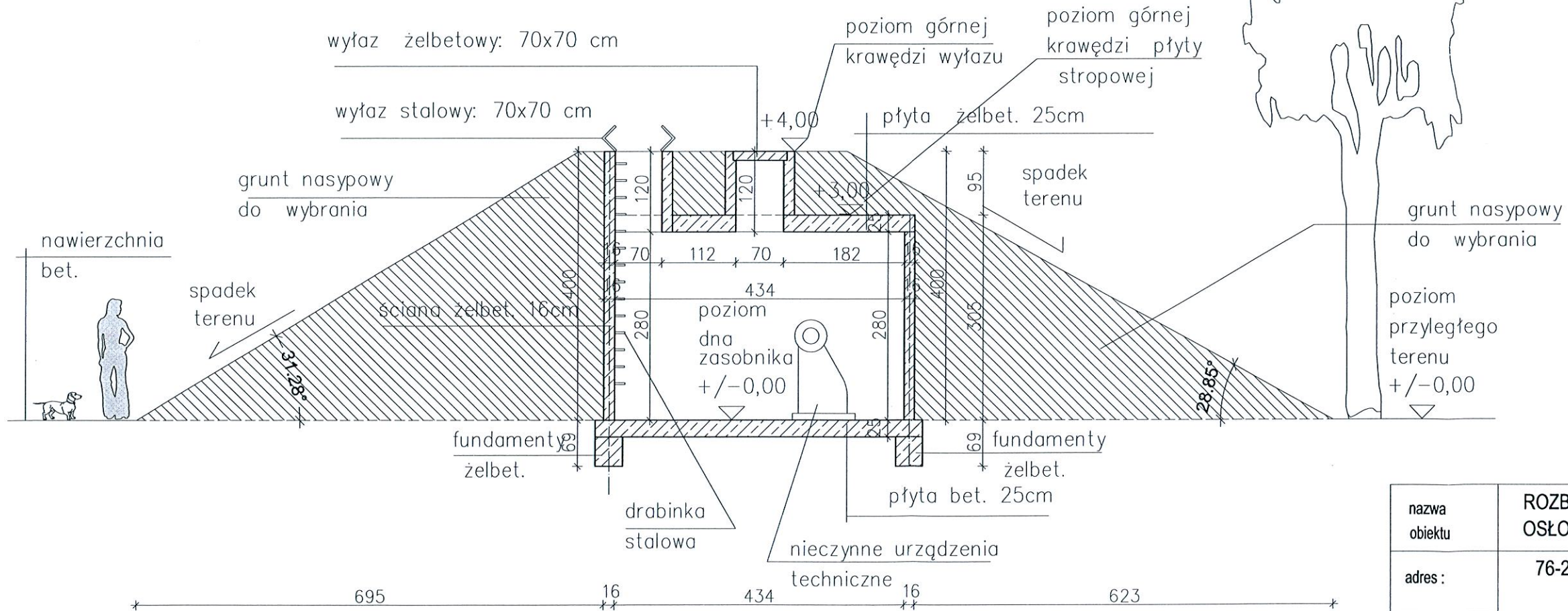
PRZEKRÓJ A-A
